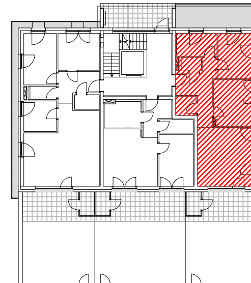
LAGE IM GEBÄUDE B2 ERDGESCHOSS
